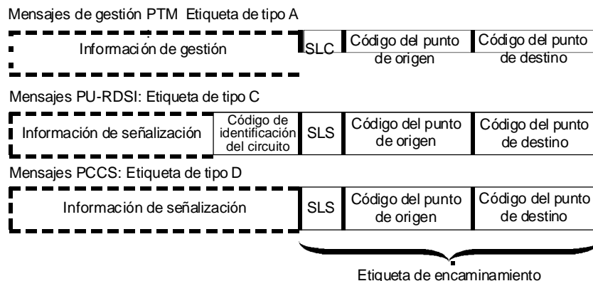
FIGURA 10.- Tipos de etiqueta de mensajes de SS7.
