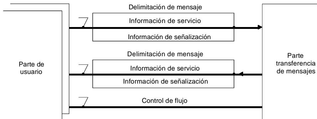
FIGURA 16.- Interfaz funcional entre la parte de transferencia de mensaje y las partes de usuario.
