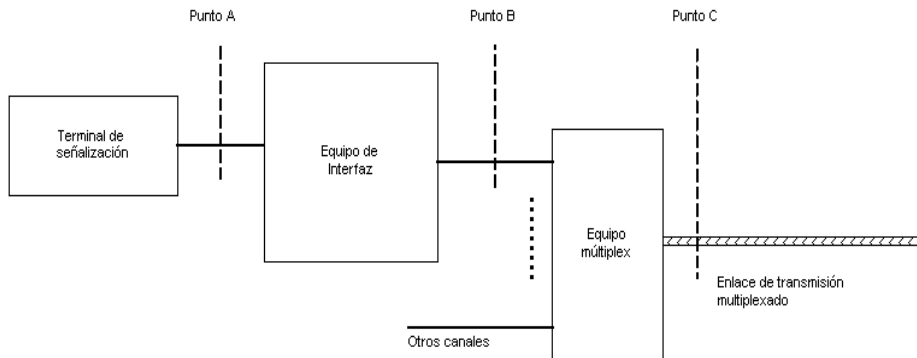
b) Ejemplo 2.- Enlace de datos de señalización (digital o analógico) mediante equipo de interfaz
