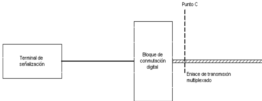
a) Ejemplo 1.- Enlace de datos de señalización digital mediante un bloque de conmutación digital
