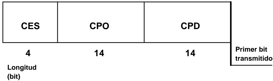
FIGURA 34.- Estructura normalizada de la etiqueta.
