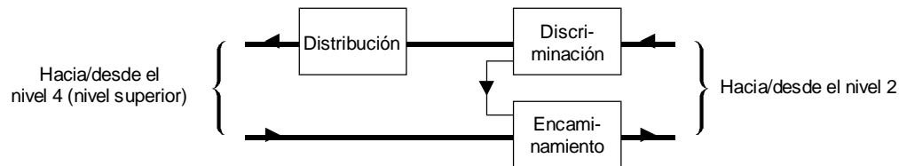
FIGURA 25.- Encaminamiento, discriminación y distribución de mensajes.
