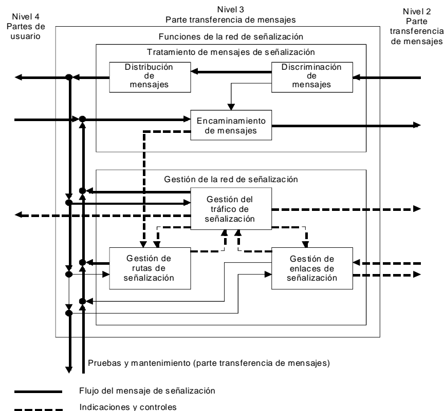
FIGURA 24.- Funciones de la red de señalización.
