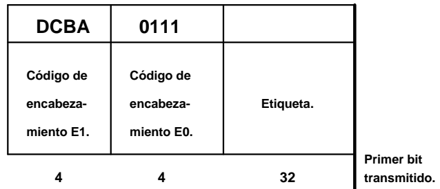
FIGURA 41.- Mensaje de reanudación de tráfico autorizada.
