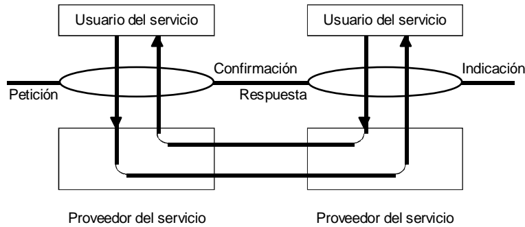
FIGURA 7.- Tipos de primitivas de servicio.
