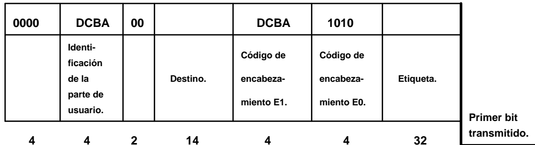
FIGURA 42-C.- Mensaje de parte de usuario indisponible.
