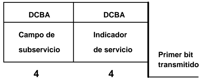
FIGURA 33.- Octeto de información de servicio.
