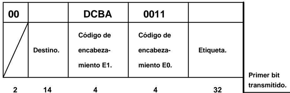
FIGURA 42-B.- Mensaje de transferencia controlada.
