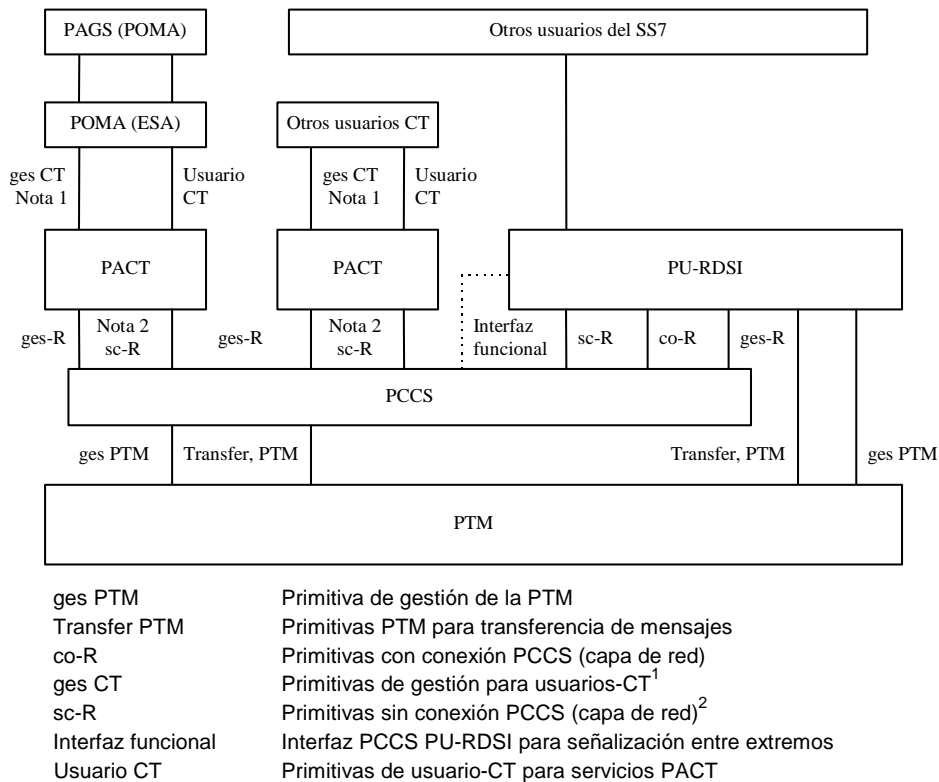
FIGURA 8.- Visión global de las primitivas utilizadas entre elementos funcionales del SS7.
