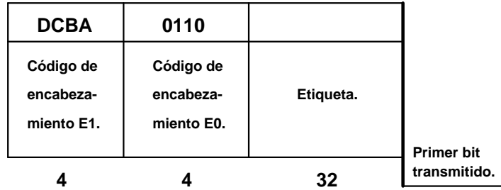
FIGURA 40-A.- Mensaje de inhibición por el sistema de administración.
