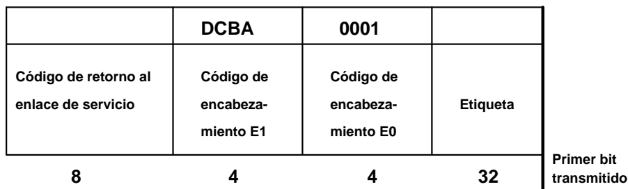
FIGURA 36.- Mensaje de retorno al enlace de servicio.
