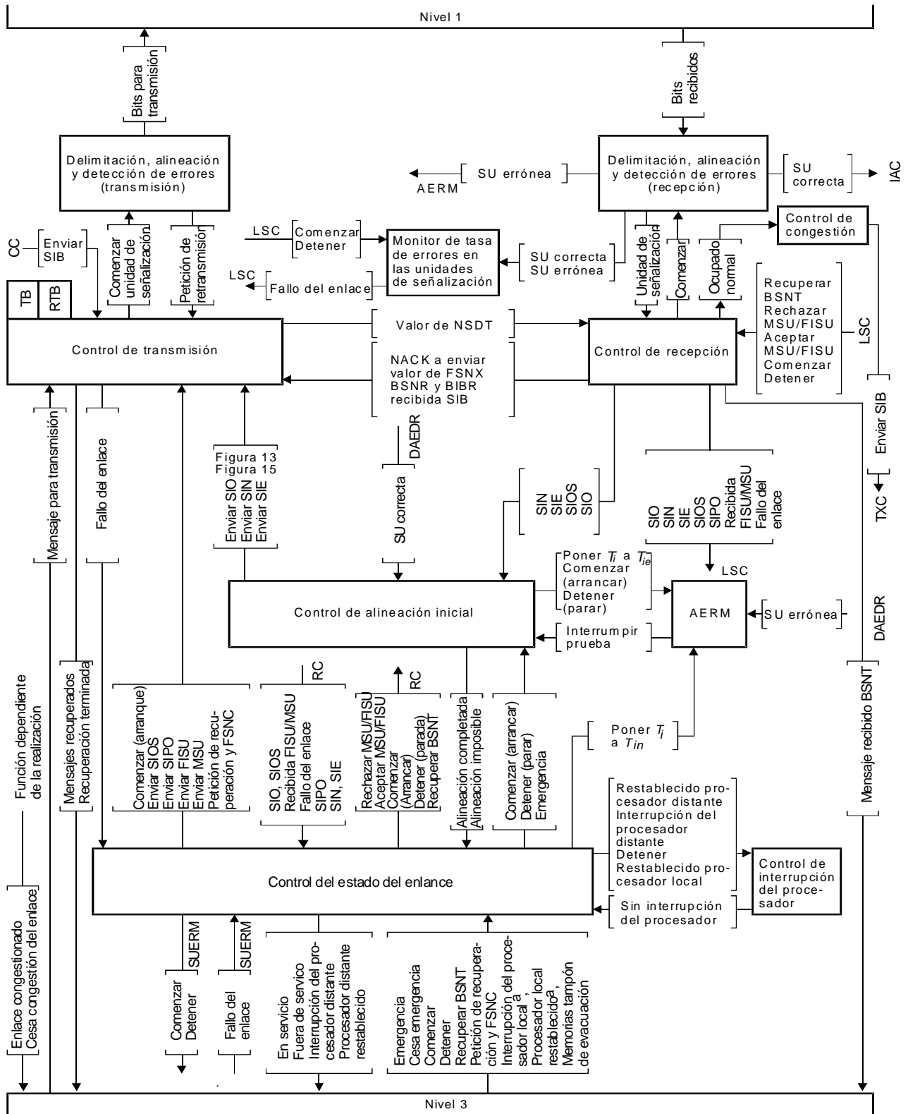
a) Sólo para la opción nacional de retención de interrupción del procesador. En este diagrama se han utilizado nombres de mensajes abreviados (es decir, se han omitido los códigos de origen-destino). Las temporizaciones utilizadas en esta figura se encuentran en 4.4.12
