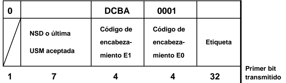
FIGURA 35.- Mensaje de paso a enlace de reserva.
