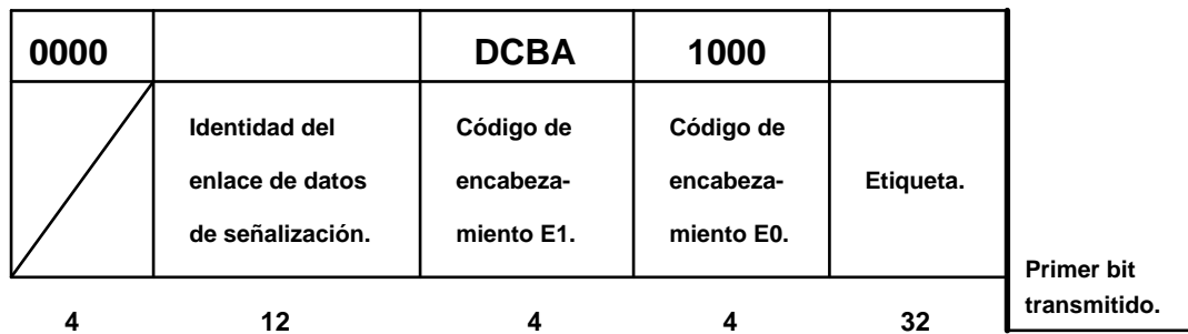
FIGURA 42.- Orden de conexión de enlace de datos de señalización.
