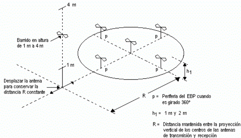
Figura A.4.- Polarización horizontal y vertical
