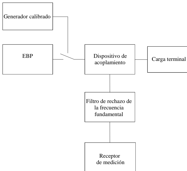
Figura 4.- Configuración de montaje para la medición de la potencia de emisiones no esenciales aplicada a la terminal de la antena
