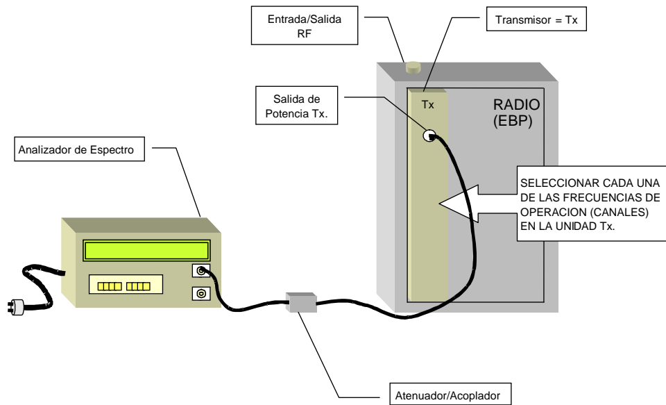
Figura 2.- Configuración para frecuencia de operación, separación entre canales y tolerancia de frecuencia
