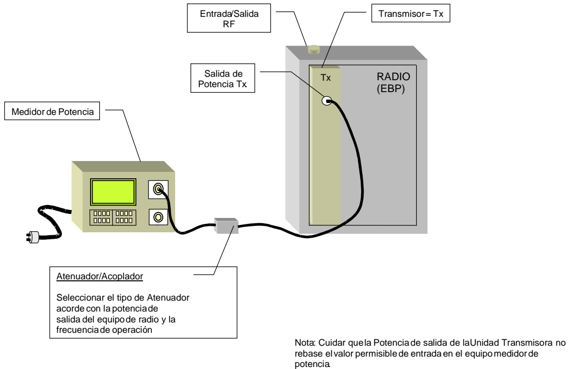
Figura 6.- Configuración para potencia media
